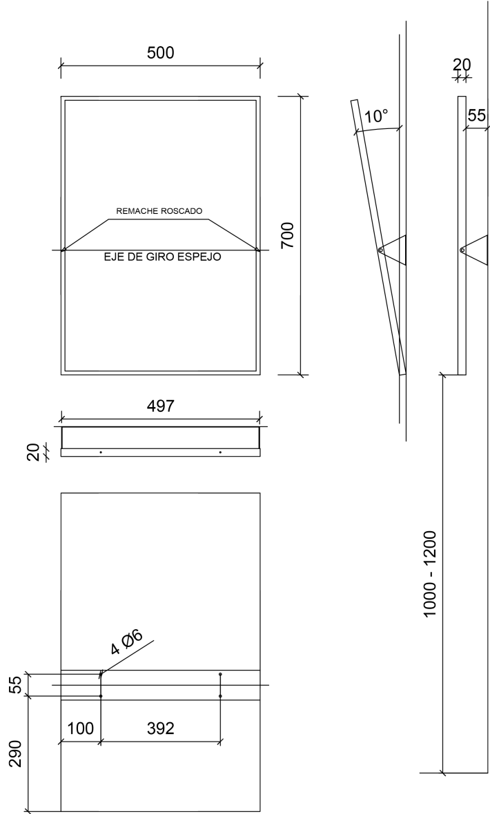
DETALLE FIJACIÓN PARED
